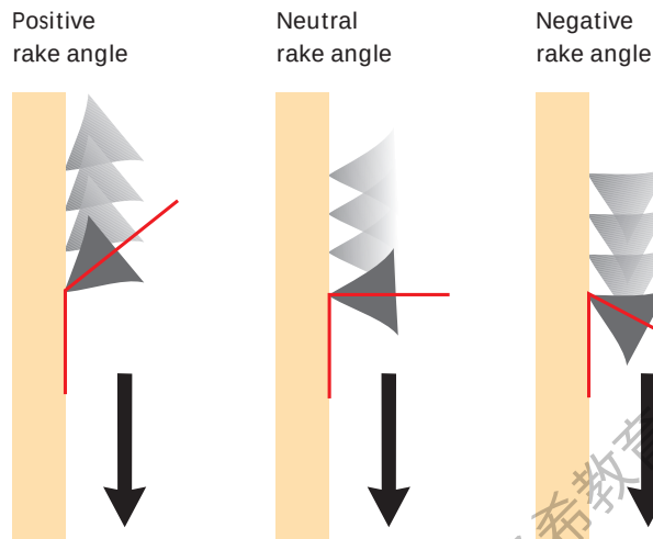
Fig. 11.20 Rake angles.
